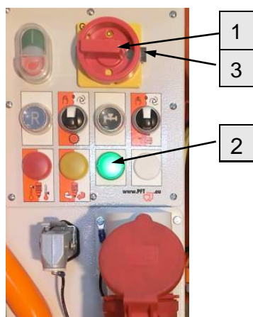
Рис. 40: Включение
