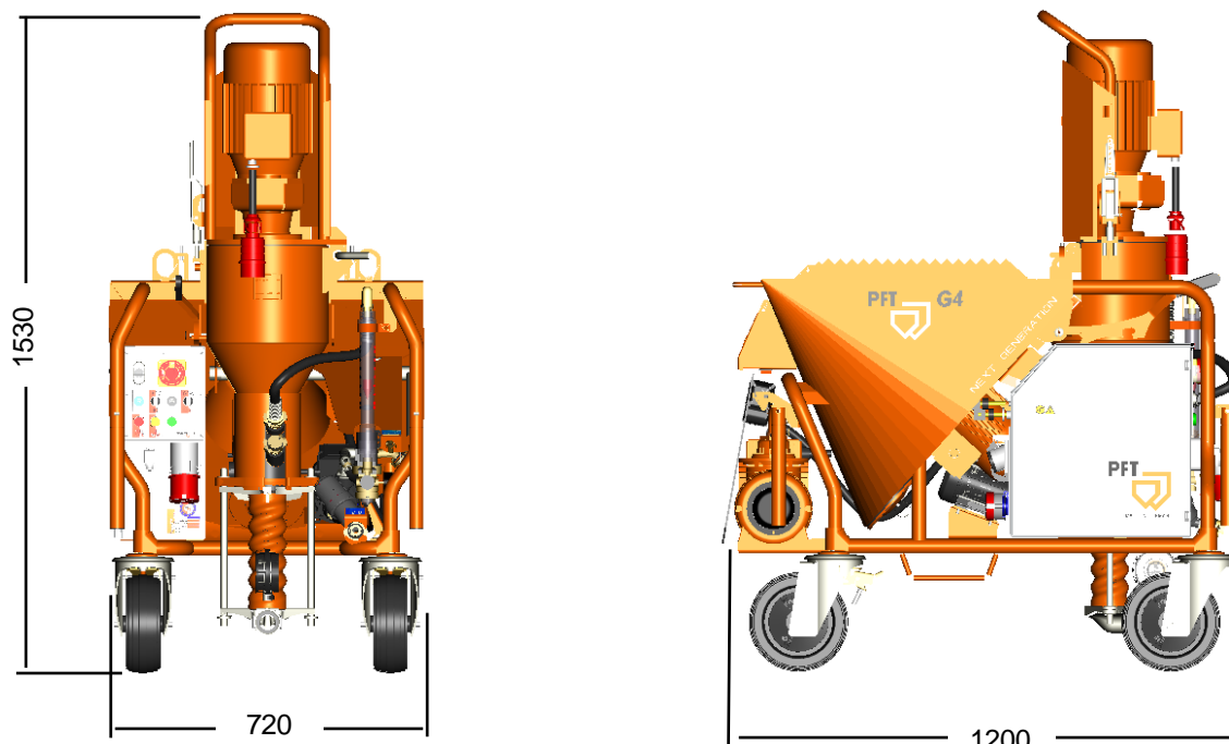
Рис. 2: Габаритный чертеж
