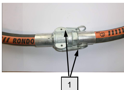
Рис. 74: Разъединение рукава
