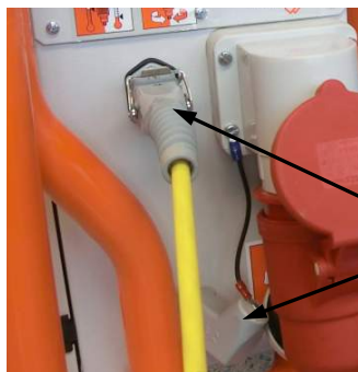
Рис. 66: Дистанционное управление
