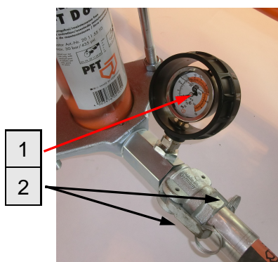
Рис. 78: Давление раствора на „0 бар“.
