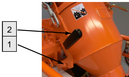
Рис. 88: Откидывание смесительной башни
