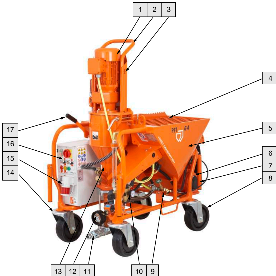
Рис. 5: Обзор узлов
