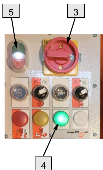
Рис. 70: Блокировка от повторного запуска
