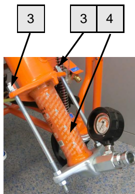
Рис. 89: Замена насоса
