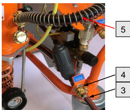
Рис. 37: Подключение воды
