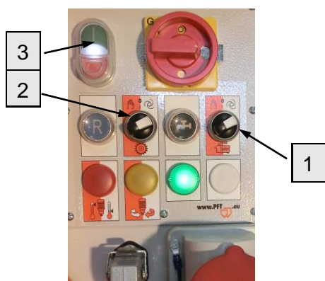
Рис. 51: Включение
