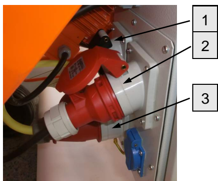
Рис. 35: Электрические подключения
