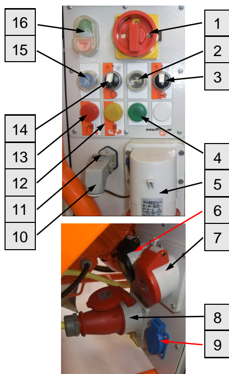
Рис. 7: Распределительный шкаф
