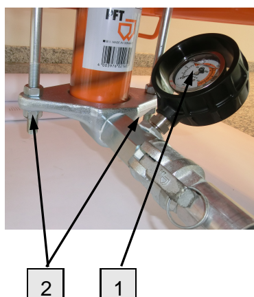
Рис. 69: Проверка давления раствора
