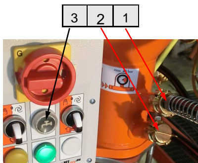
Рис. 43: Увлажнение
