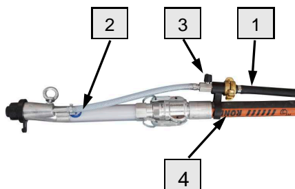
Рис. 58: Растворный пистолет
