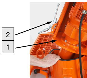
Рис. 84: Опускание упорного буртика
