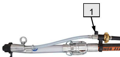
Рис. 63: Закрывание воздушного крана
